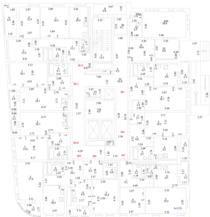
2 этаж
