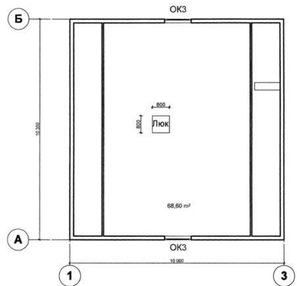
План чердака
